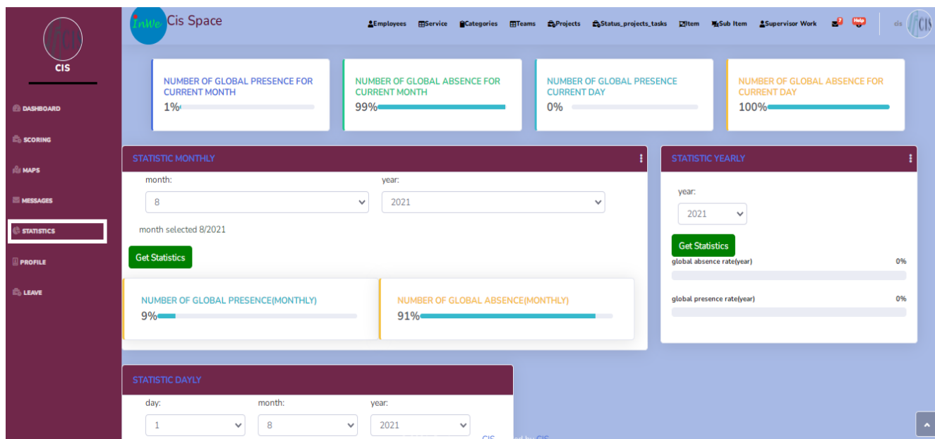
Figure 9:Statistique globale.
